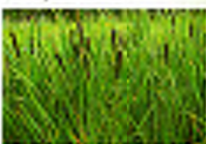
Рогоз узколистный
